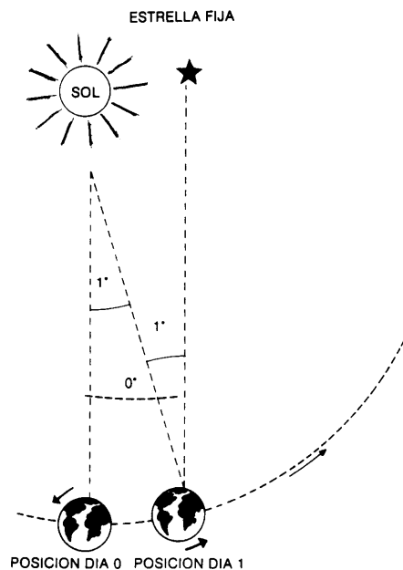
FIGURA 14 MEDICION DEL DIA TERRESTRE: TRASLACION DE 1° DE LA TIERRA EN UN DIA
