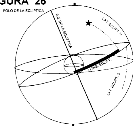
FIGURA 26 LATITUD Y LONGITUD ECLIPTICAS. POLO DE LA ECLIPTICA
