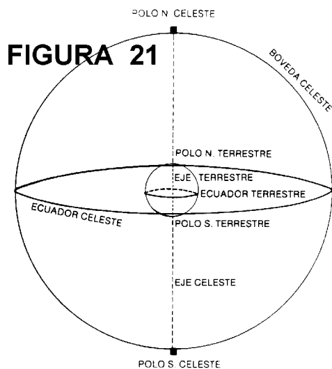
FIGURA 21 EJE, POLOS, ECUADOR Y BOVEDA
