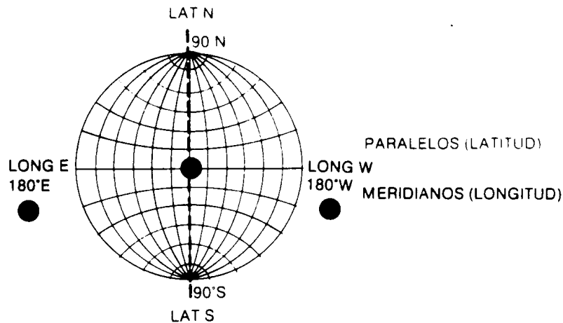
FIGURA 12 LATITUD Y LONGITUD TERRESTRES
