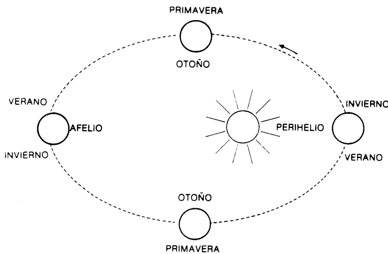
FIGURA 16 ORBITA DE LA TIERRA Y RELACION CON LAS ESTACIONES
