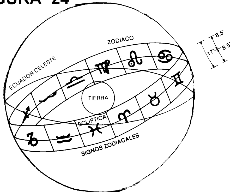
FIGURA 24 ZODIACO Y ANTERIORES
