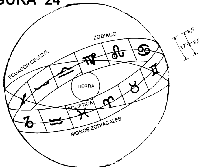
FIGURA 24 ZODIACO Y ANTERIORES
