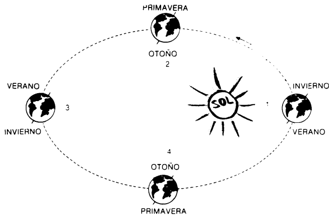
FIGURA 18 LAS 4 ESTACIONES: POSICION DEL EJE TERRESTRE EN CADA ESTACION RESPECTO AL SOL.
