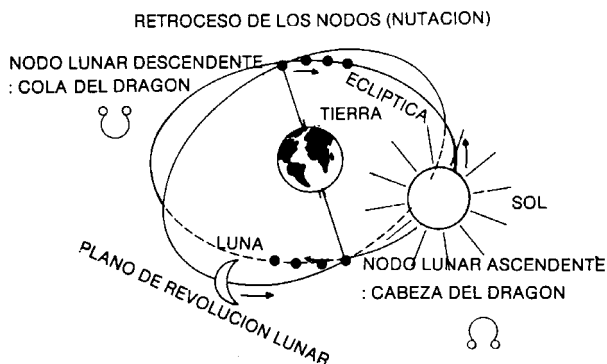
FIGURA 33 PUNTOS DE CORTE ENTRE LA ECLIPTICA Y EL PLANO DE REVOLUCION LUNAR: NODOS LUNARES. NUTACION
