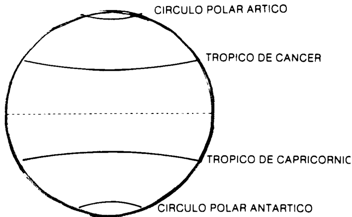
FIGURA 13 TROPICOS Y CIRCULOS POLARES
