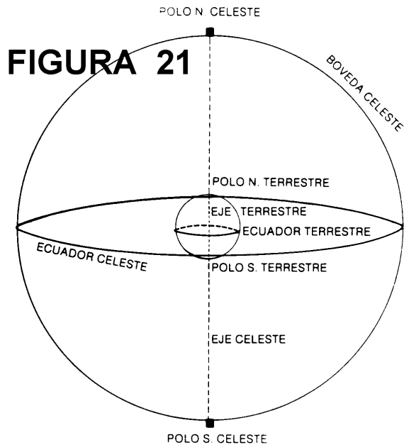
FIGURA 21 EJE, POLOS, ECUADOR Y BOVEDA
