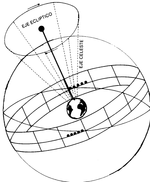
FIGURA 30 TRASLACION DEL EJE ECUATORIAL CELESTE ALREDEDOR DEL EJE ECLIP- TICO: CORTES SUCCESIVOS EN RETROCESO DE LOS EQUINOCCIOS. PRECESION EQUINOCCIAL.
