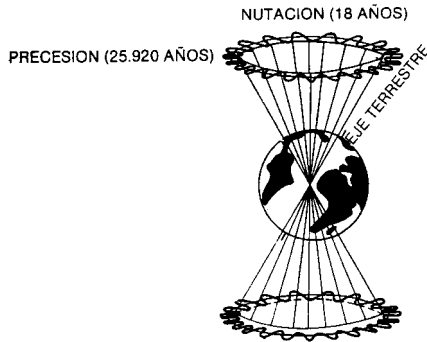
FIGURA 34 NUTACION Y PRECESION SIMULTANEAS
