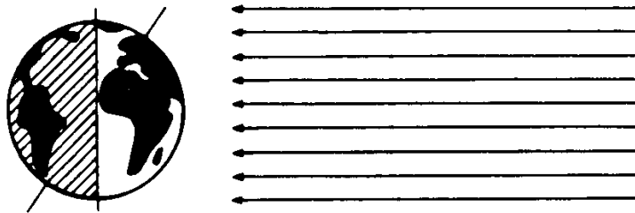
FIGURA 15 EL DIA Y LA NOCHE
