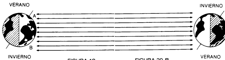
FIGURA 19 DETALLE DE LA POSICION 3 FIGURA 20-B DETALLE DE LA POSICION 1
